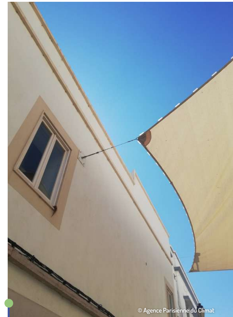
À Faro, les voiles d'ombrage sont fixées via des plaques de métal vissées aux bâtiments
